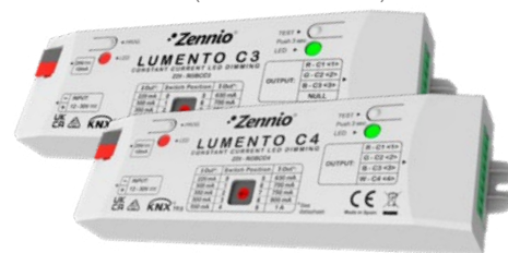
ZDI-RGBCC4 (144 x 44 x 22 mm)
